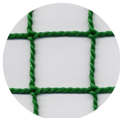
ポリエチレン 440T 36本 25mm角 無結節 グリーン
