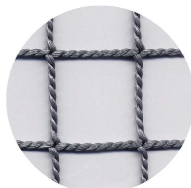
ポリエチレン 440T 36本 25mm角 無結節 シルバ-グレー
